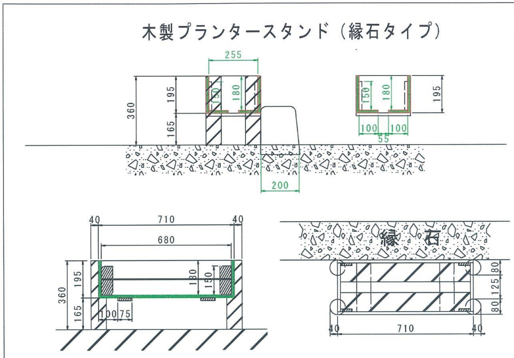
(参考) プランター構造図
